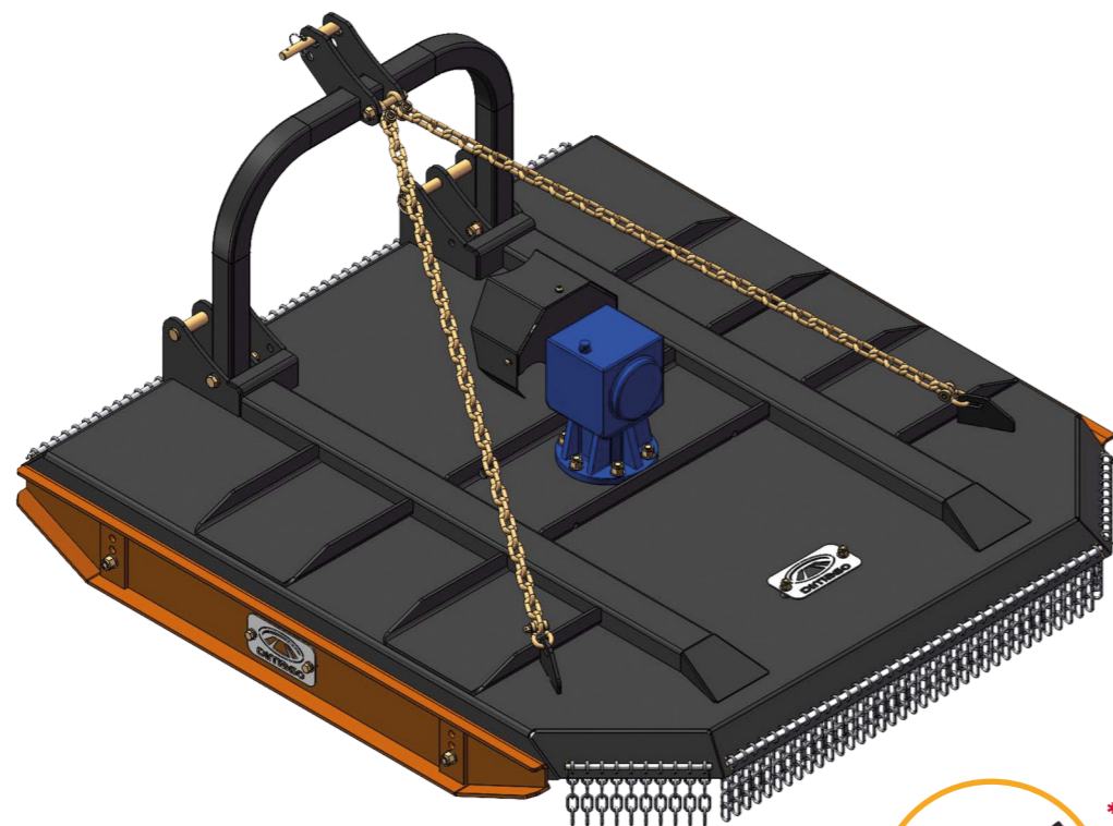
SISTEMA DE CORTE POR CUCHILLAS
